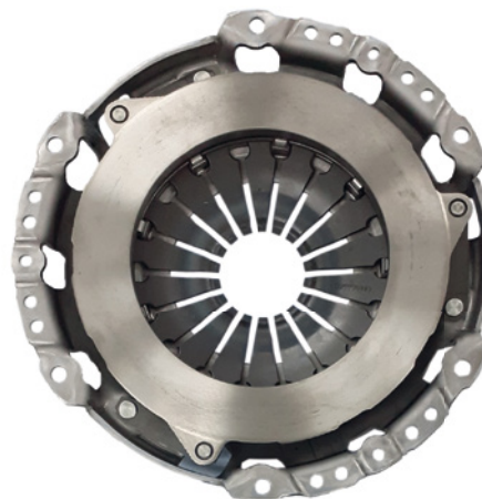
Figuur 2: Drukplaat 120 0505 10 met klein wrijvingsoppervlak diameter 200mm
